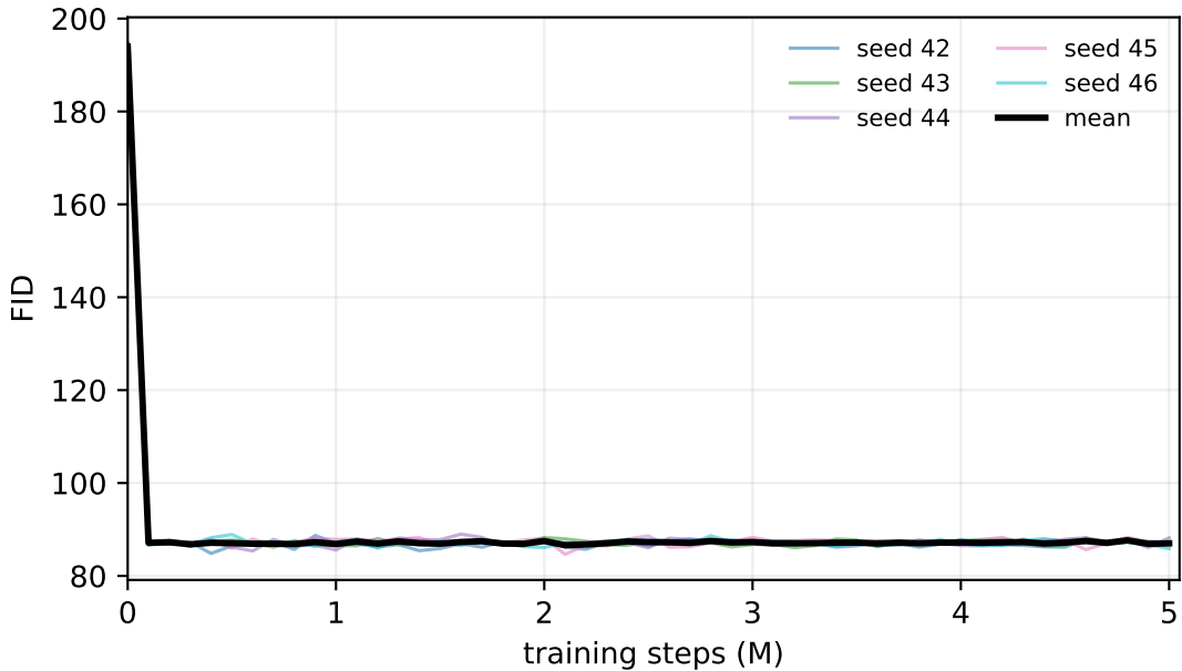
CelebA d=10
